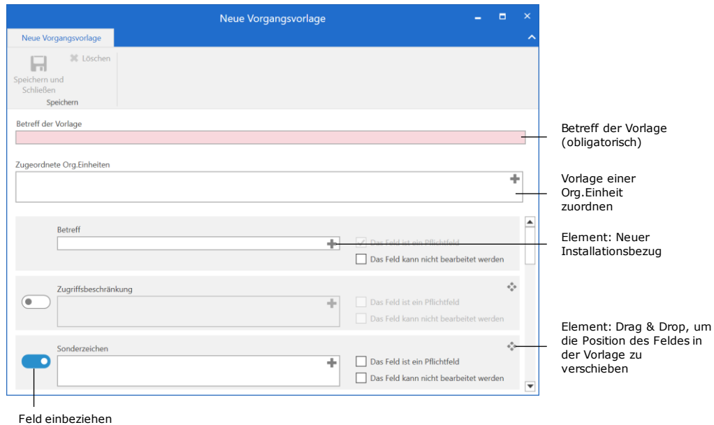
Abbildung 6: Neue Vorgangsvorlage
