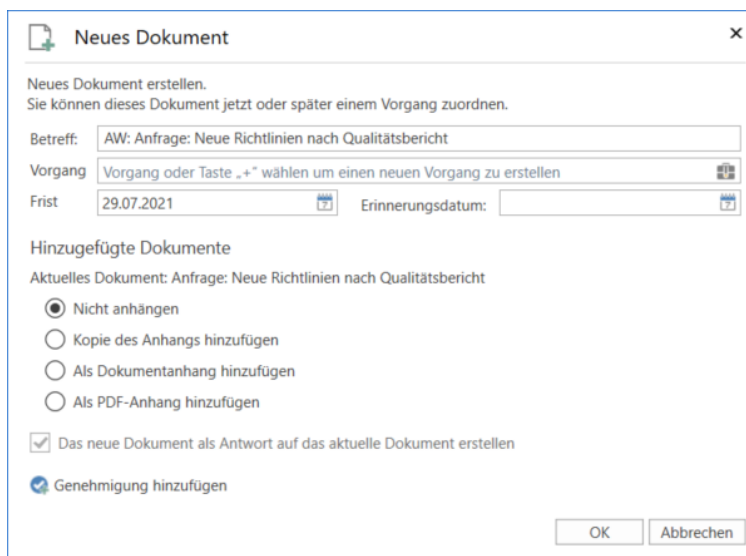
Abbildung 11: Antwortdokument erstellen
