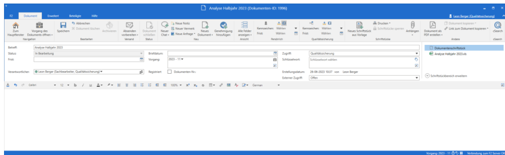
Abbildung 7: Komplettes Dokumentenfenster
