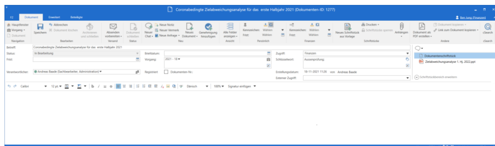
Abbildung 8: Komplettes Dokumentenfenster
