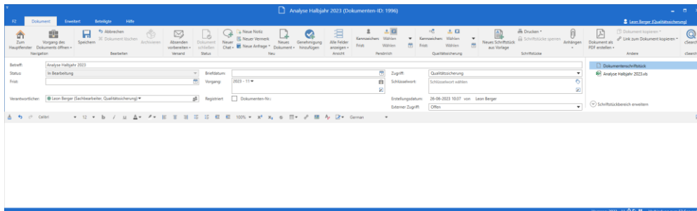
Abbildung 8: Komplettes Dokumentenfenster
