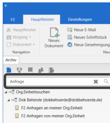
Abbildung 4: Ausschnitt des Hauptfensters. Das Filterfeld über der Listenübersicht ist markiert. Text wurde eingegeben und die Listenübersicht zeigt nur Suchlisten an, die mit dem Text übereinstimmen
