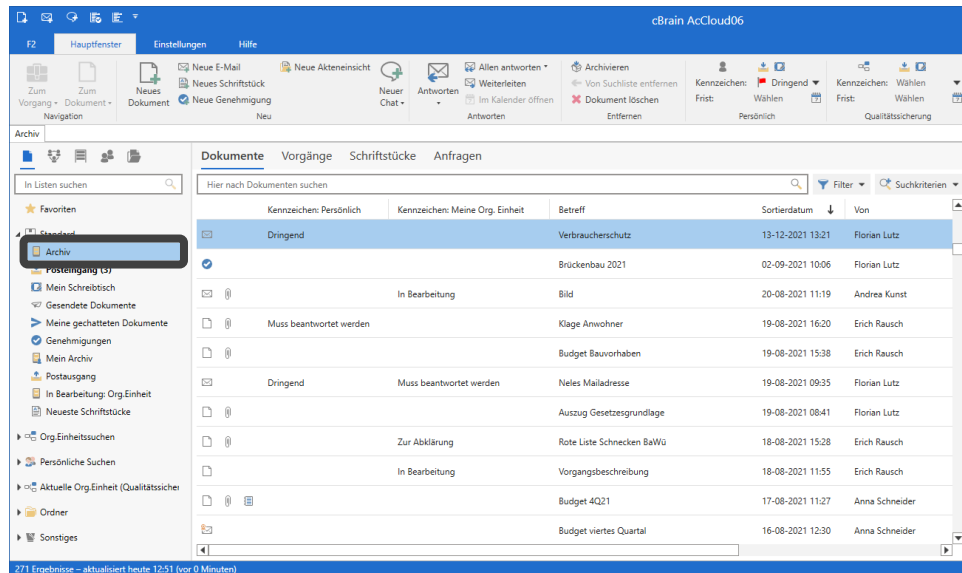
Abbildung 6: Ausschnitt des Hauptfensters. In der Listenübersicht ist die Suchliste „Archiv“ markiert und ihr Inhalt ist in der Ergebnisliste dargestellt
