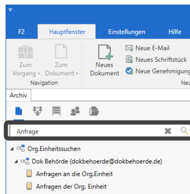
Abbildung 4: Ausschnitt des Hauptfensters. Das Filterfeld über der Listenübersicht ist markiert. Text wurde eingegeben und die Listenübersicht zeigt nur Suchlisten an, die mit dem Text übereinstimmen
